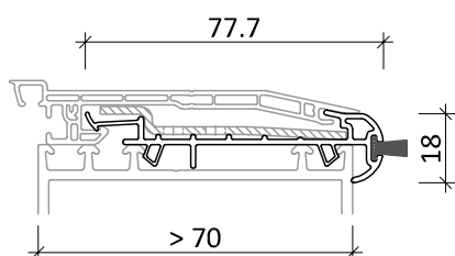
Basisprofil „A“ 77,7 x 18 mm
