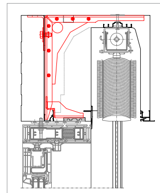
ROKA-TOP® 2 SHADOW
