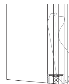
Unterschieneinstellung für Z 73 / Z 90 / Z 93
