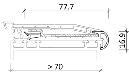
Basisprofil „D“ 77,7 x 16,9 mm
