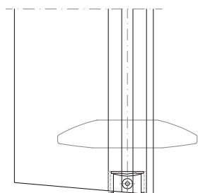
Unterschieneinstellung für F 60 / F 80 und C 60 / C 80
