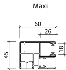
Führungsschiene ALU 60 x 45 mm
