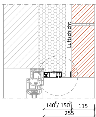
SHADOW-TG 87,5 mm für Klinkermauerwerk
