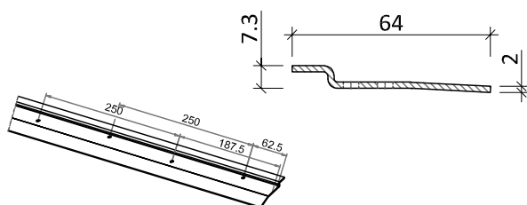
Verstärkungsseisen VARIANT 64 x 7,3 x 2 mm
