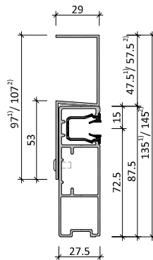
FSCH 27-87 mit ALU-Zusatzprofil für Klinkermauerwerk
