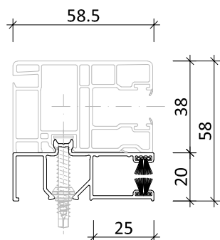
Führungsschiene Aluminium-Insektenschiene 58,5 x 20 mm (Schwarz oder Weiß) passend zu Führungsschiene PVC 58 x 38 mm
