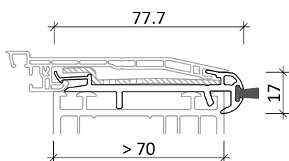
Basisprofil „B“ 77,7 x 17 mm
