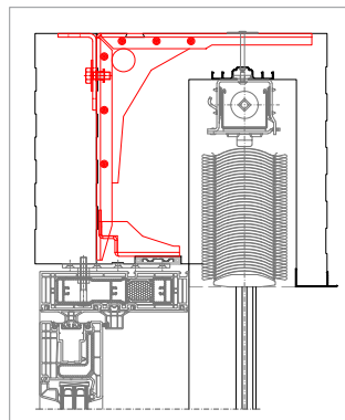
ROKA-TOP® 1 SHADOW
