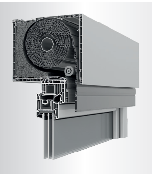
ROKA-VARIANT 2 Insektenschutz
