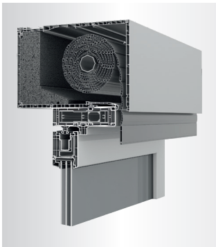
ROKA-VARIANT 2 HST
