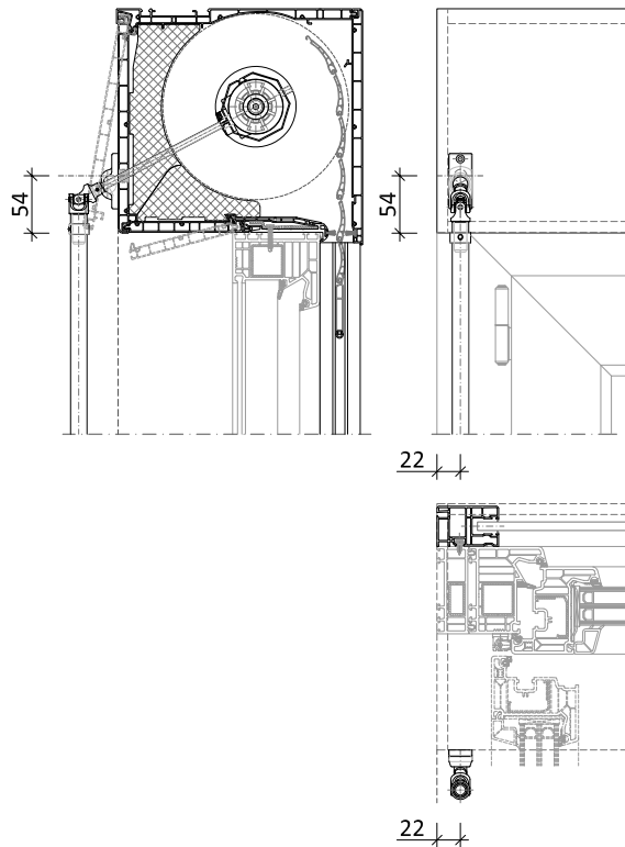
Kurbelbedienung innen Kurbelausgang A
