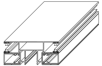
Doppelführungsschiene ALU 96,8 x 41 mm
