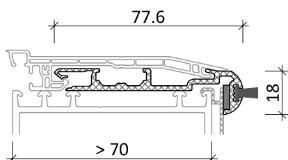
Basisprofil „E“ 77,6 x 18 mm
