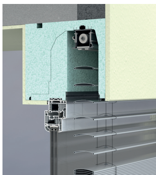
Putz (Monolithisch)
