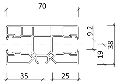
Doppel-Führungsschiene PVC 70 x 38 mm Mini mit Dichtung Grau
