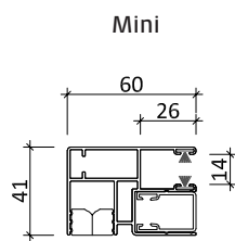
Führungsschiene ALU 60 x 41 mm
