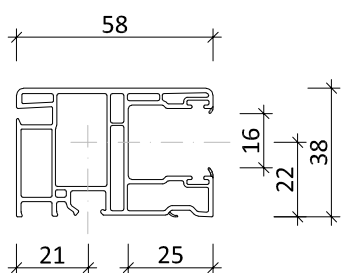
Führungsschiene PVC 58 x 38 mm Maxi mit Dichtung Grau
