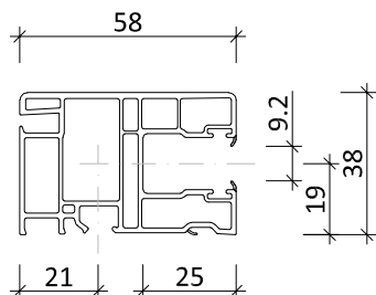
Führungsschiene PVC 58 x 38 mm Mini mit Dichtung Grau
