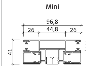
Doppelführungsschiene ALU 96,8 x 41 mm
