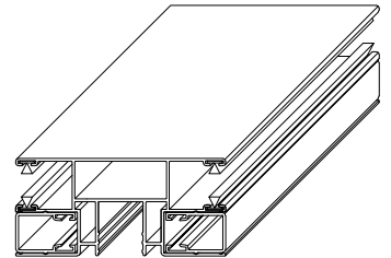
Doppelführungsschiene ALU 96,8 x 45 mm
