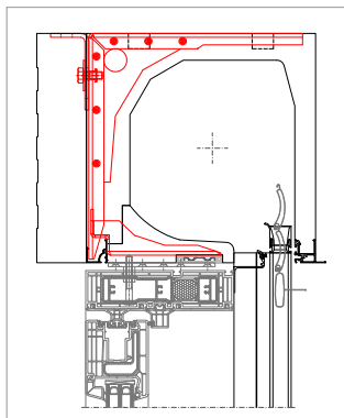
ROKA-TOP® 2 RG
