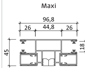
Doppelführungsschiene ALU 96,8 x 45 mm
