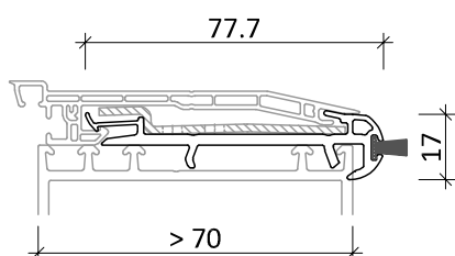
Basisprofil „C“ 77,7 x 17 mm
