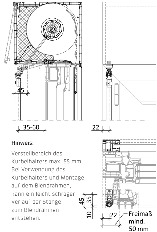
Kurbelbedienung unten Kurbelausgang B
