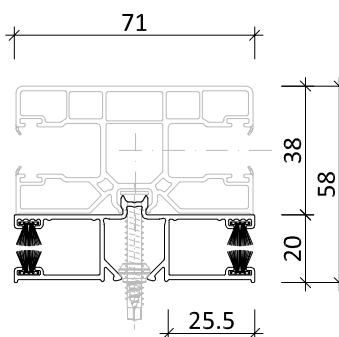
Doppel-Führungsschiene Aluminium-Insektenschiene 71 x 20 mm (Schwarz oder Weiß) passend zu Doppel-Führungsschiene PVC 70 x 38 mm
