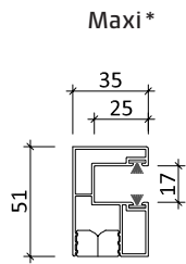
Führungsschiene ALU 35 x 51 mm
