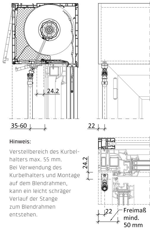
Kurbelbedienung unten Kurbelausgang C
