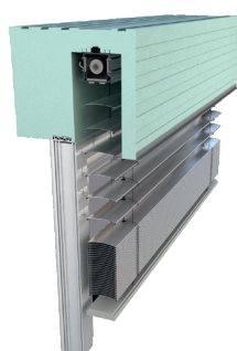
ROKA-TOP® 1 SHADOW
