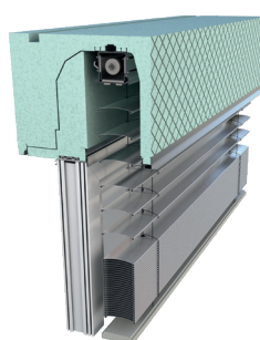
ROKA-TOP® 2 SHADOW
