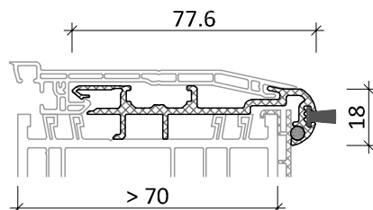
Basisprofil „F“ 77,6 x 18 mm
