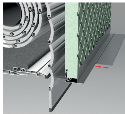
Eingeschäumte Abschlusschienen (Zusatzprofile optional)
