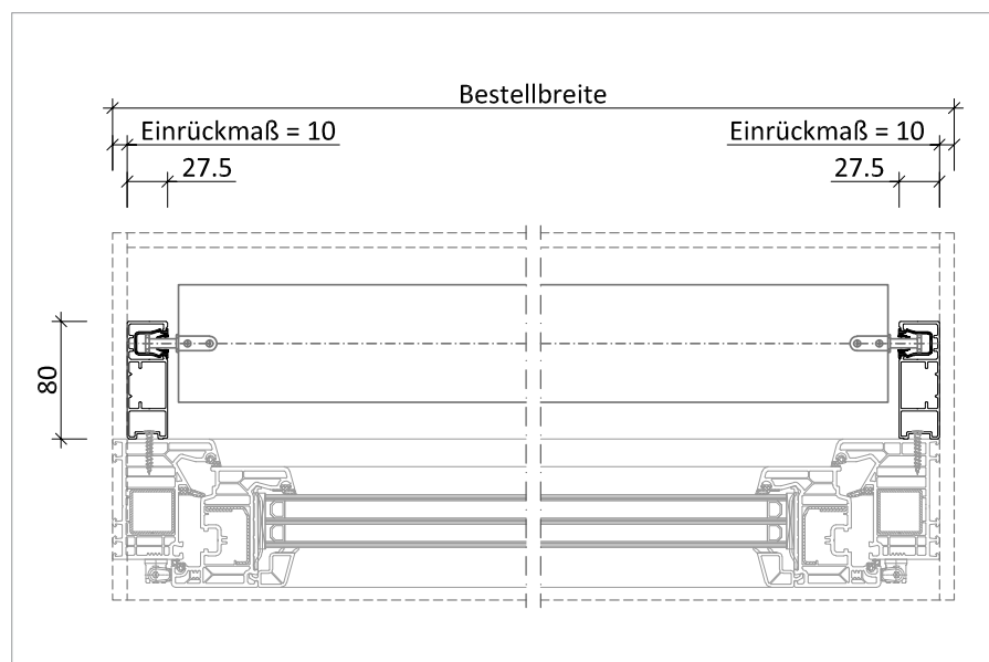
Führungsschiene ROKA-VARIANT 2 Raffstore
