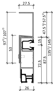
Grundschiene 87,5 mm (Standard) mit ALU-Zusatzprofil für Klinkermauerwerk
