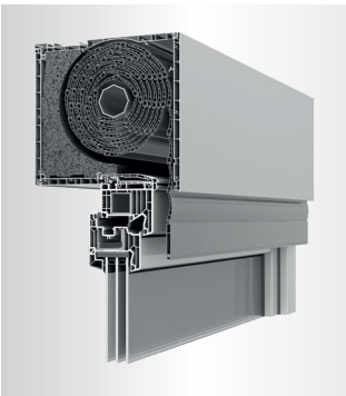
ROKA-VARIANT 2
