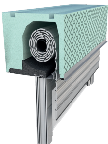
ROKA-TOP® 2 RG
