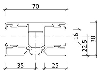
Doppel-Führungsschiene PVC 70 x 38 mm Maxi mit Dichtung Grau
